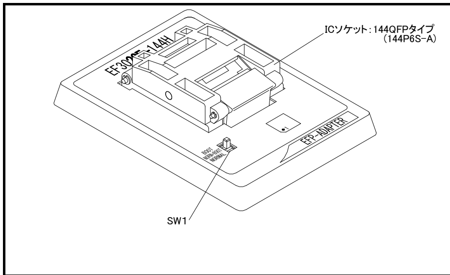
図1. 1 EF3022F-144H外形図
