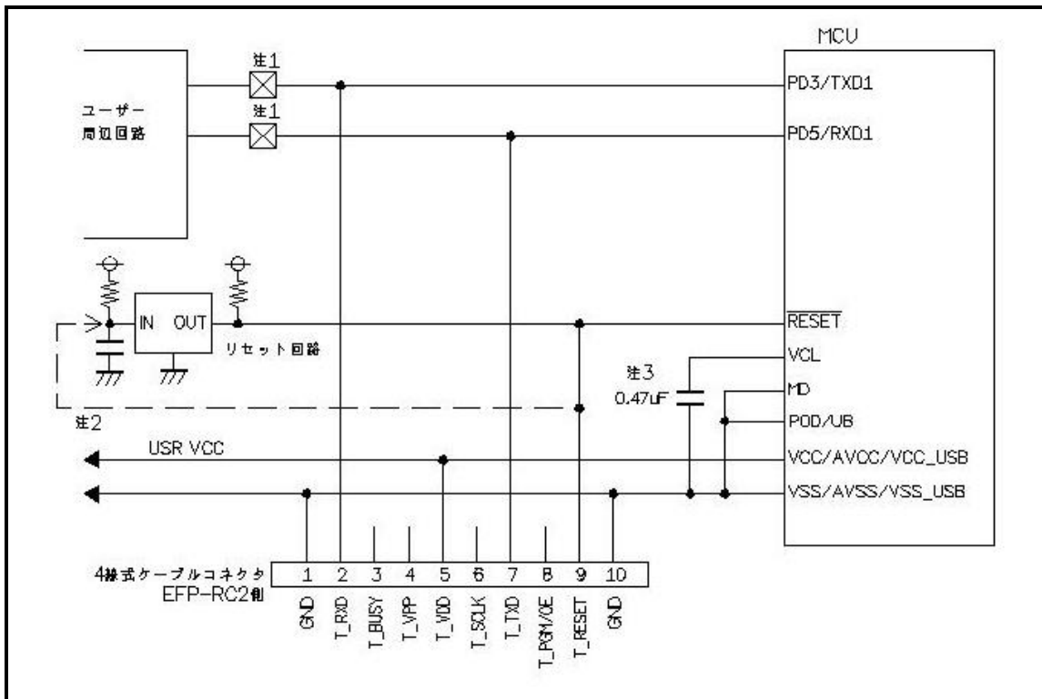
図5.1 ユーザーターゲット推奨回路図
