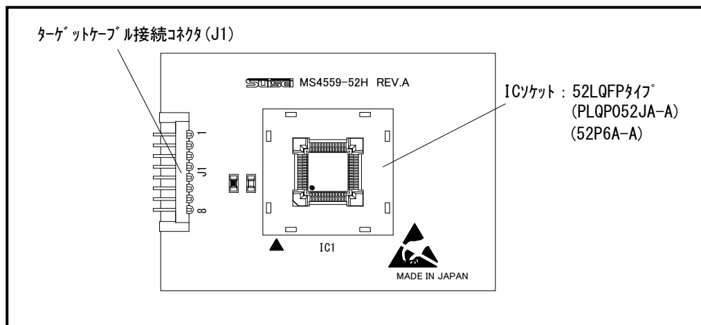
図 1.1 MS4559-52H 外観図
