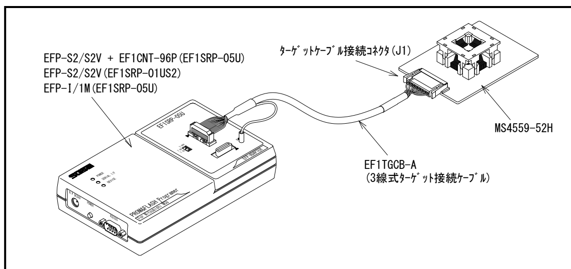
図 2. 1 EF 1 T G C B - A (3線式ターゲット接続ケーブル) との接続
